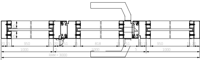
Horizontalschnitt 1-flüglige Stahl-Lofttür mit Seitenteilen
