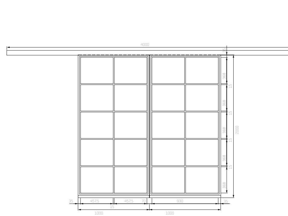
2-flüglige Stahl-Lofttür
