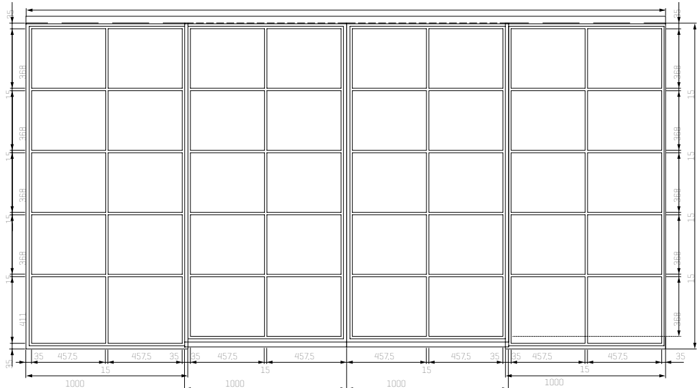
2-flüglige Stahl-Lofttür mit Seitenteilen
