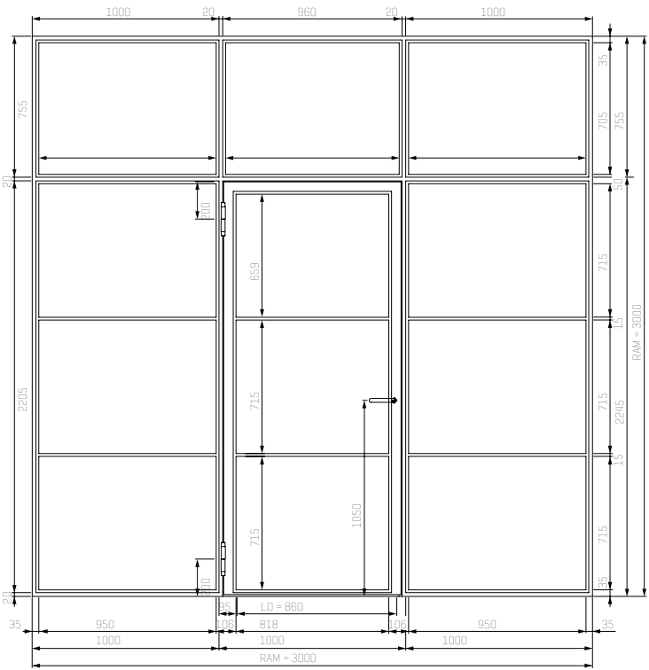
1-flüglige Stahl-Lofttür mit Seitenteilen und Oberlicht
