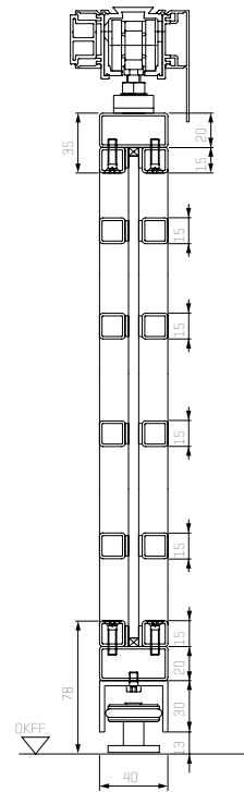
Vertikalschnitt 1-flüglige Stahl-Lofttür
