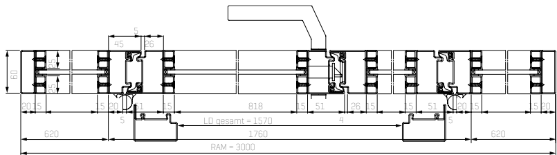
Horizontalschnitt 2-flüglige Stahl-Lofttür mit Seitenteilen
