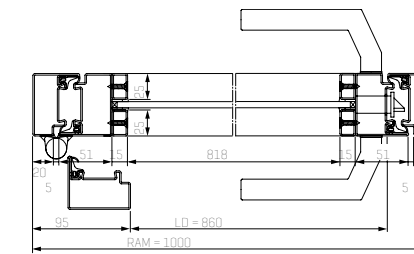
Horizontalschnitt 1-flüglige Stahl-Lofttür
