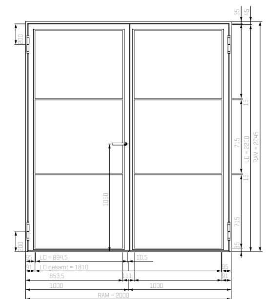
2-flüglige Stahl-Lofttür
