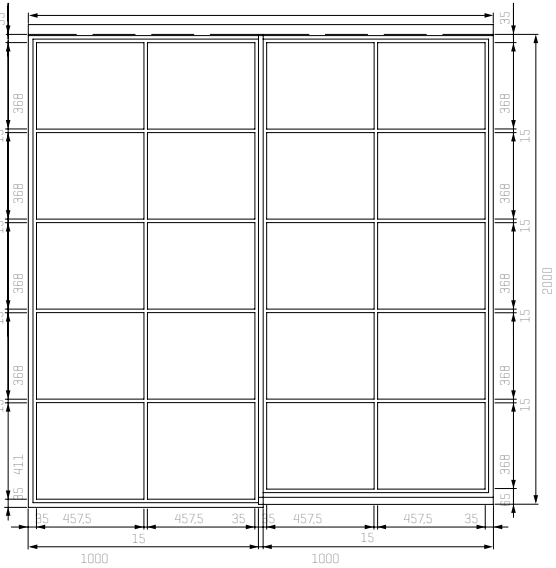
2-flüglige Stahl-Lofttür mit Seitenteil
