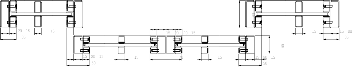
Horizontalschnitt 2-flüglige Stahl-Lofttür mit Seitenteilen
