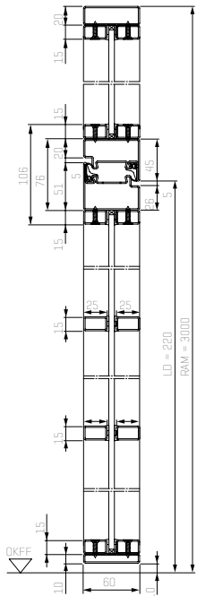
Vertikalschnitt 2-flüglige Stahl-Lofttür mit Oberlicht
