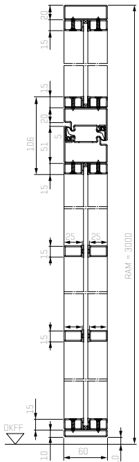
Vertikalschnitt 1-flüglige Stahl-Lofttür mit Oberlicht
