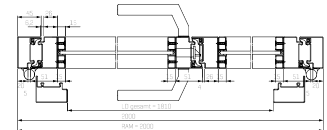
Horizontalschnitt 2-flüglige Stahl-Lofttür
