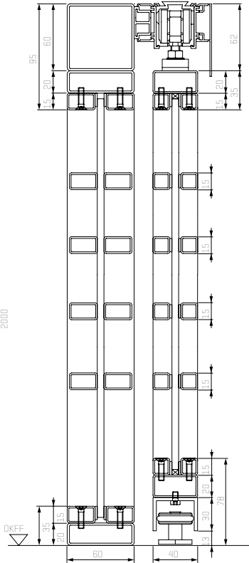
Vertikalschnitt 2-flüglige Stahl-Lofttür mit Seitenteilen
