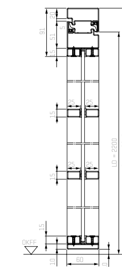
Vertikalschnitt 1-flüglige Stahl-Lofttür
