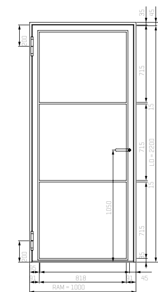
1-flüglige Stahl-Lofttür
