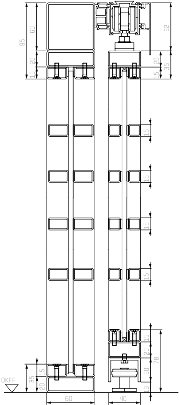
Vertikalschnitt 2-flüglige Stahl-Lofttür mit Seitenteil
