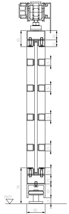
Vertikalschnitt 2-flüglige Stahl-Lofttür
