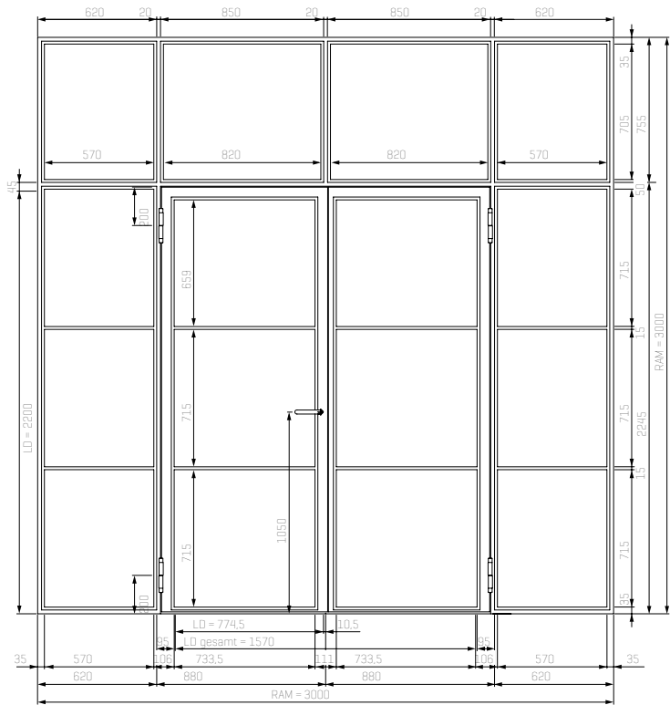
2-flüglige Stahl-Lofttür mit Seitenteilen und Oberlicht
