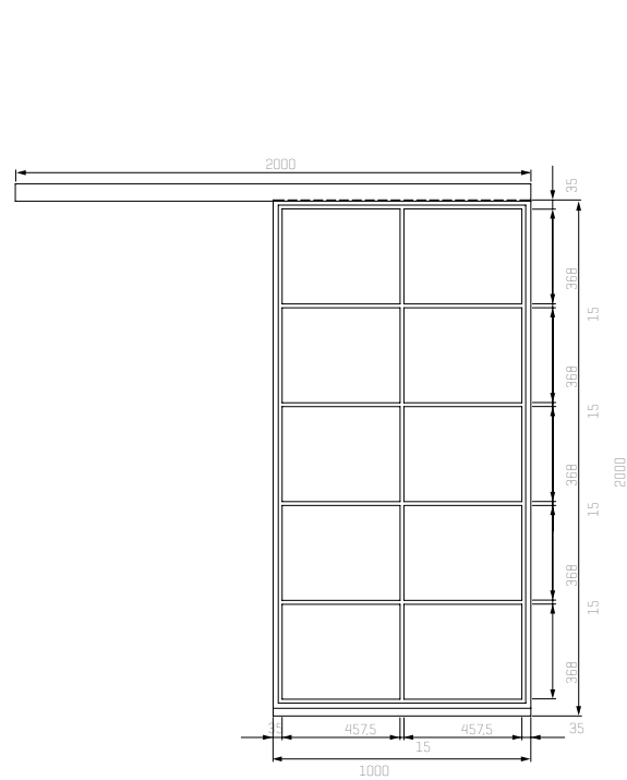
1-flüglige Stahl-Lofttür
